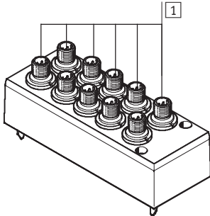
1 Connettore M12x1, perno, a 5 poli
