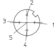
1 Connettore M12x1, perno, a 5 poli
