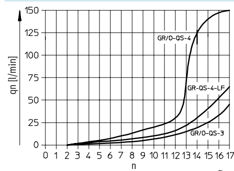
Portata normale qn a 6 bar → 0 bar in funzione del numero di giri della vite n Attacco a innesto QS-3/QS-4
