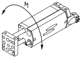
Zulässiges Drehmoment M in Abhängigkeit von der Hublänge l (an der Frontplatte)
