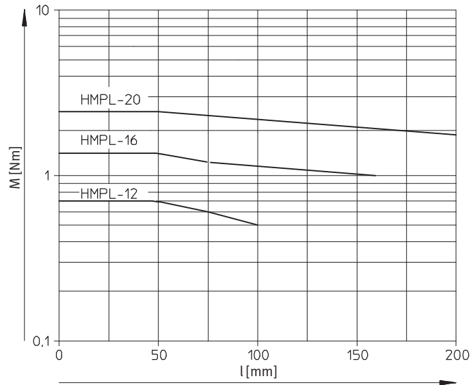
Zulässiges Drehmoment M in Abhängigkeit von der Hublänge l (an der Frontplatte)
