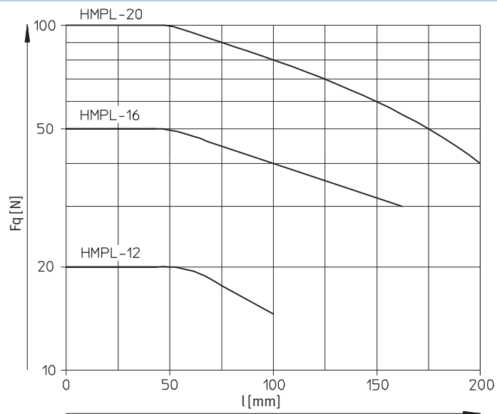
Zulässige Nutzlast F_q in Abhängigkeit von der Hublänge l (an der Frontplatte)
