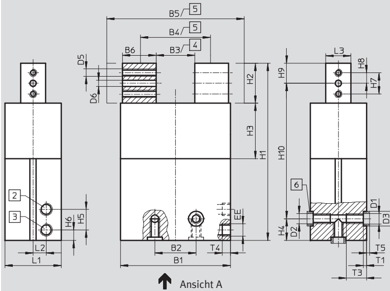
Ansicht A HGP-06-A
