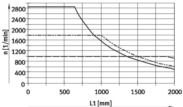
Max. Drehzahl n in Abhängigkeit von der Nennlänge L1
