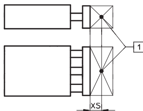
1 Nutzlastschwerpunkt
