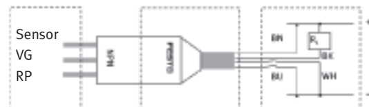
Kabelbaum zur VADMI
