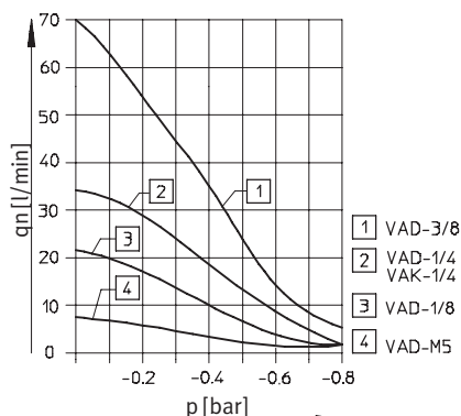
Saugvermögen q_n in Abhängigkeit vom Vakuum p
