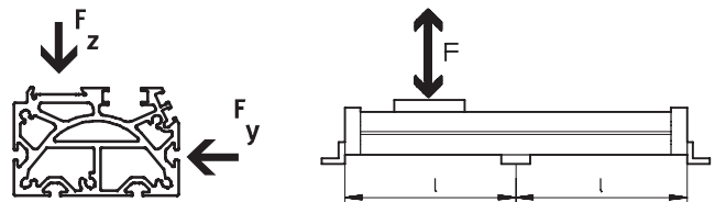
Kraft F_z
