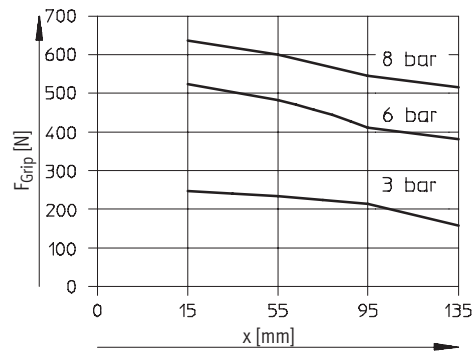
HGPL-40-80-A
