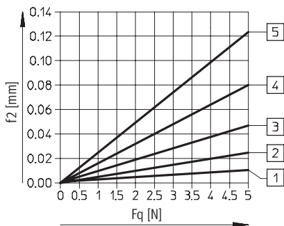
Piston \varnothing 6 mm
