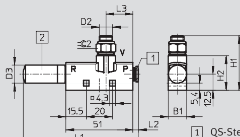
1 QS-Steckanschluss 2 Schalldämpfer
