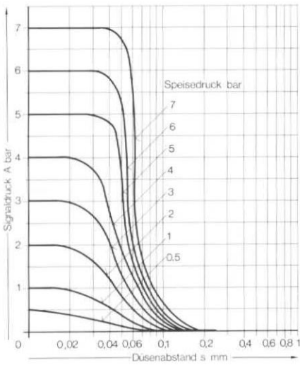
Typ SD-2
