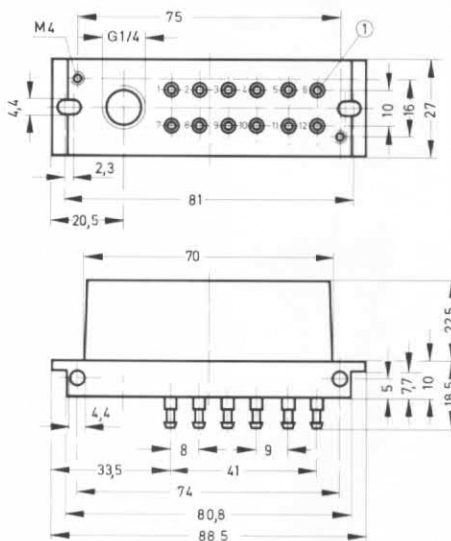
① Stecknippel für Kunststoffschlauch
