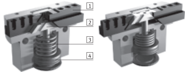
Greifer geschlossen
