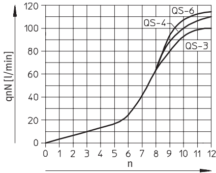
Normalnennendurchfluss q_{nN} [l/min] bei 6 bar \rightarrow 5 bar in Abhängigkeit der Spindelumdrehungen n Einschraubgewinde M5
