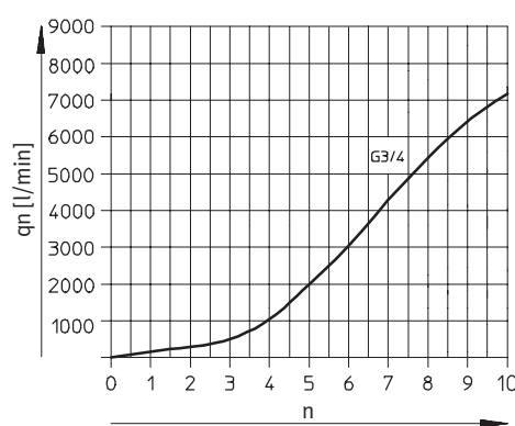
Einschraubgewinde G3/4
