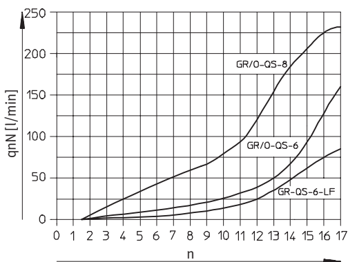
Steckanschluss QS-6/QS-8
