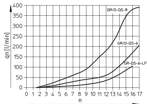
Steckanschluss QS-6/QS-8
