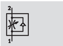
Zuluft-Drossel-Rückschlag GRLZ
