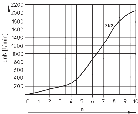
Einschraubgewinde G1/2
