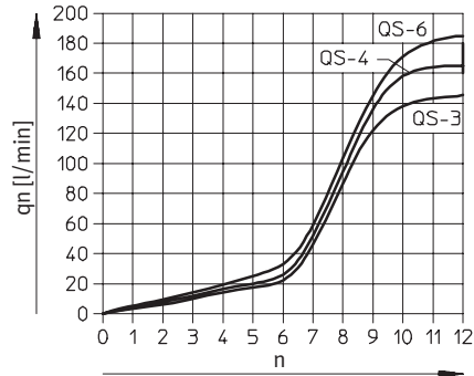
Normaldurchfluss q_n bei 6 bar \rightarrow 0 bar in Abhängigkeit der Spindelumdrehungen n Einschraubgewinde M5
