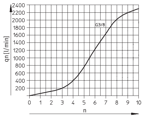
Normaldurchfluss q_n bei 6 bar \rightarrow 0 bar in Abhängigkeit der Spindelumdrehungen n Einschraubgewinde G3/8
