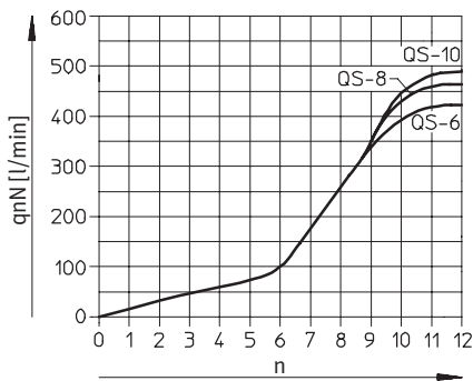
Einschraubgewinde G\frac{1}{8} mit Durchfluss MF
