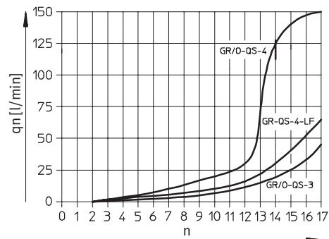
Normaldurchfluss q_n bei 6 bar \rightarrow 0 bar in Abhängigkeit der Spindelumdrehungen n Steckanschluss QS-3/QS-4
