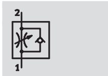
Zuluft-Drossel-Rückschlag GRLZ
