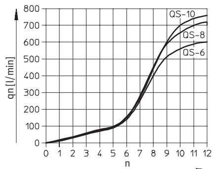
Einschraubgewinde G\frac{1}{4}
