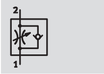
Abluft-Drossel-Rückschlag GRLA
