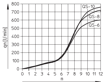
Einschraubgewinde G\frac{1}{8} mit Durchfluß MF
