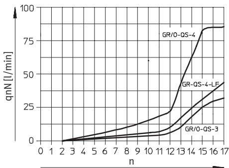
Normalnenndurchfluss q_{nN} bei 6 bar \rightarrow 5 bar in Abhängigkeit der Spindelumdrehungen n Steckanschluss QS-3/QS-4
