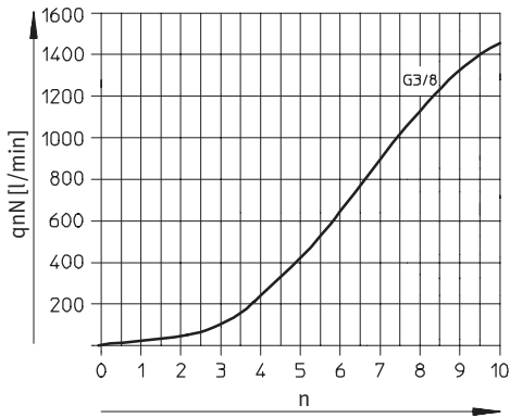
Normalnenndurchfluss q_{nN} bei 6 bar \rightarrow 5 bar in Abhängigkeit der Spindelumdrehungen n Einschraubgewinde G3/8
