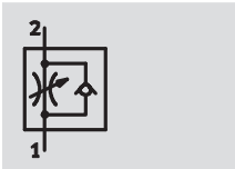
Zuluft-Drossel-Rückschlag GRLZ/GRGZ
