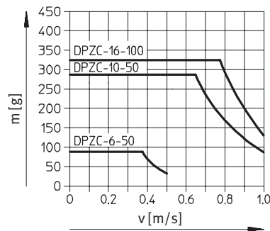
Kugelumlaufführung KF
