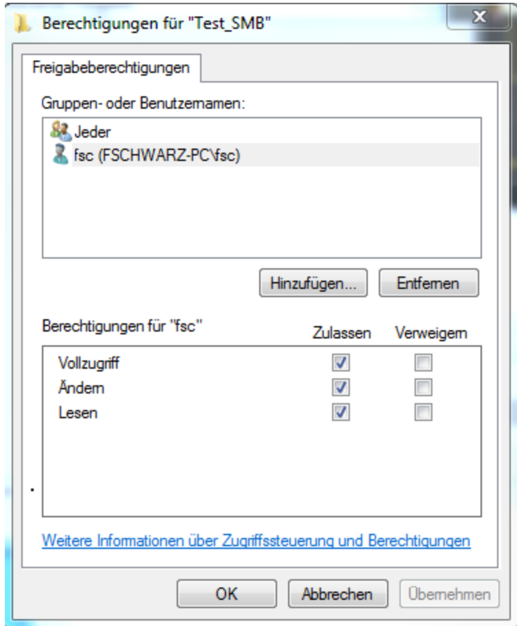
Abbildung 165: Berechtigungen vergeben
