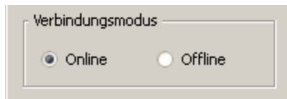
Abbildung 113: Abbildung, Verbindungsmodus
