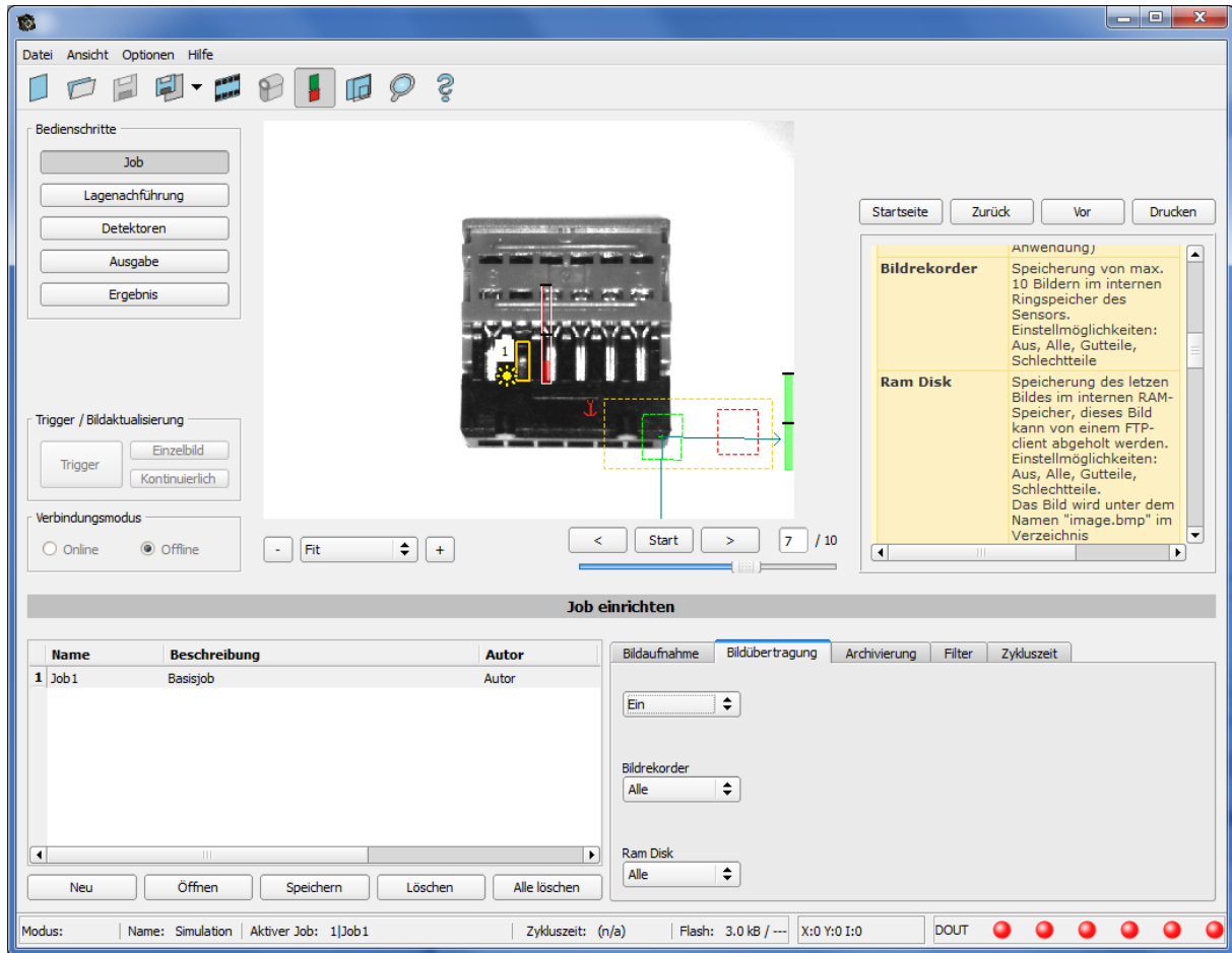
Abbildung 169: Ram Disk
