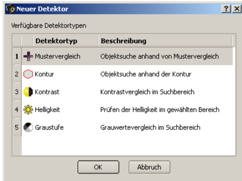
Abbildung 32: Detektorliste Objektsensor
